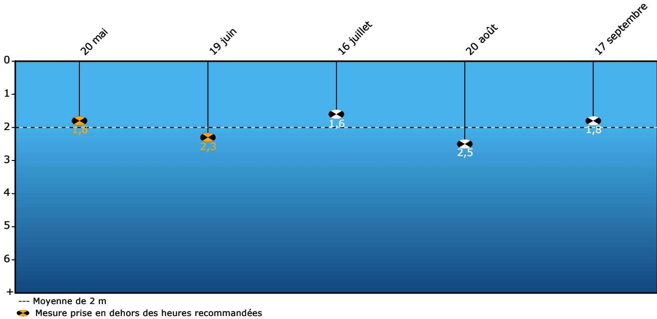
Transparence de l'eau - Été 2014 (profondeur du disque de Secchi en mètres)
