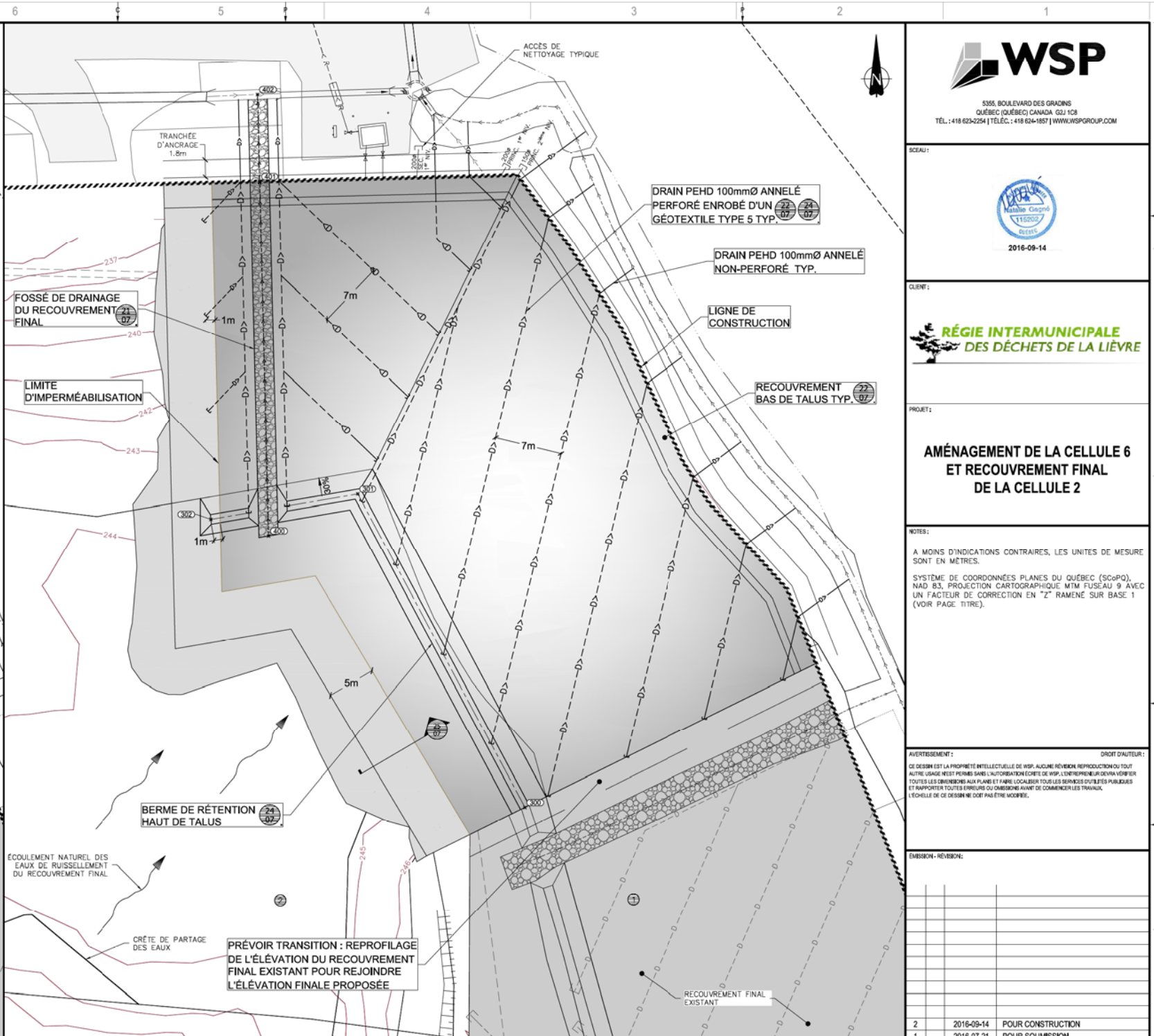
VUE EN PLAN DRAINAGE DU RECOUVREMENT FINAL
