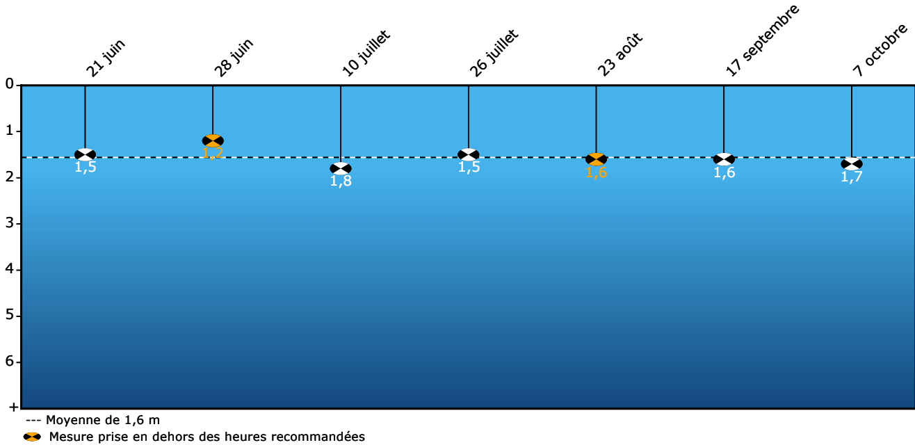
Transparence de l'eau - Été 2021 (profondeur du disque de Secchi en mètres)
