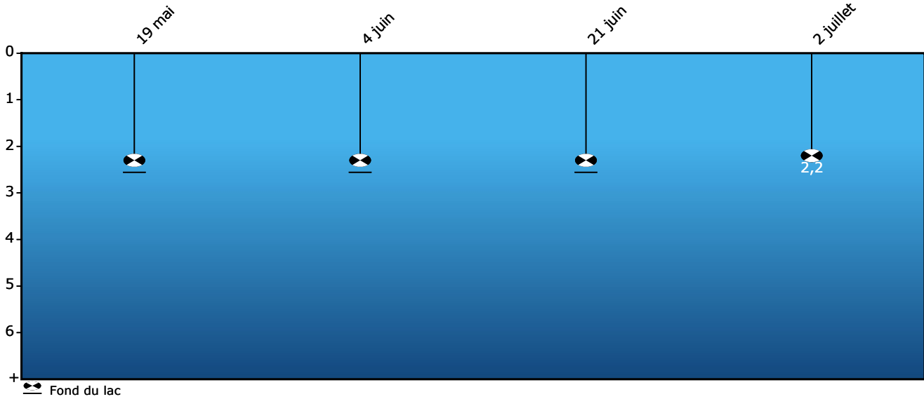
Transparence de l'eau - Été 2019 (profondeur du disque de Secchi en mètres)
