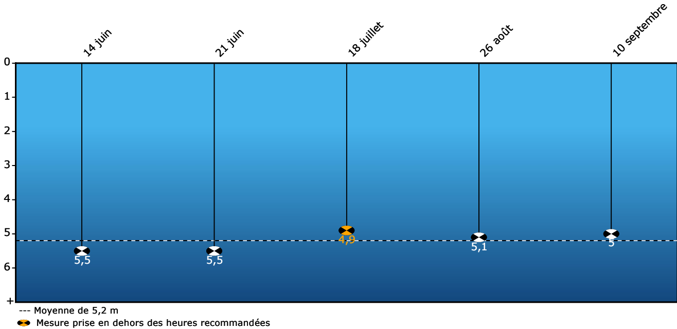
Transparence de l'eau - Été 2011 (profondeur du disque de Secchi en mètres)
